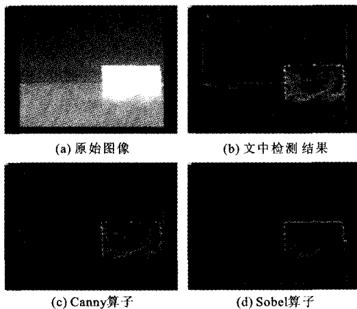
图 1 红外图像检测结果
