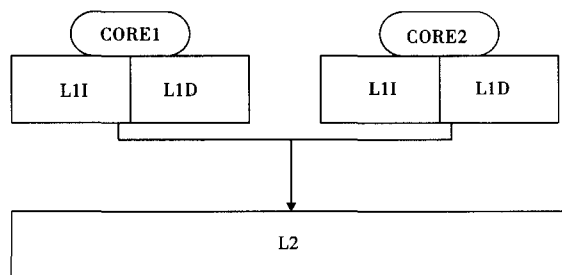
图 1 共享二级 Cache
