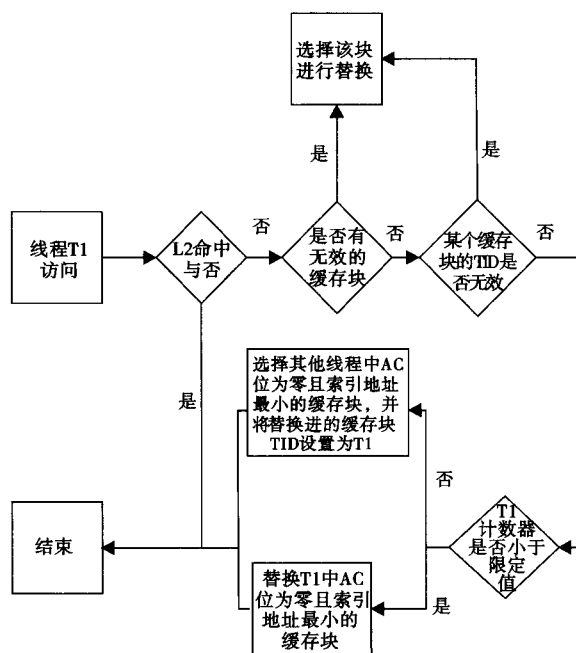
图 4 划分算法流程
