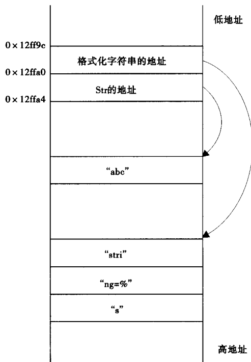
图 1 正确调用时内存情况
