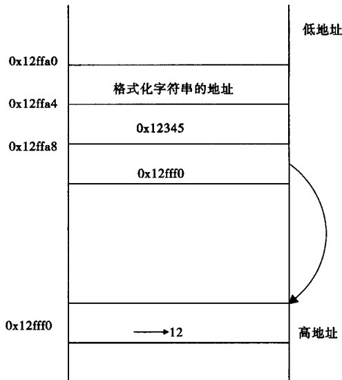
图 2 错误调用时内存情况 1
