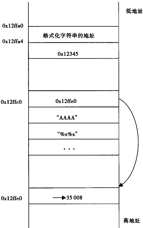
图 3 错误调用时内存情况 2
