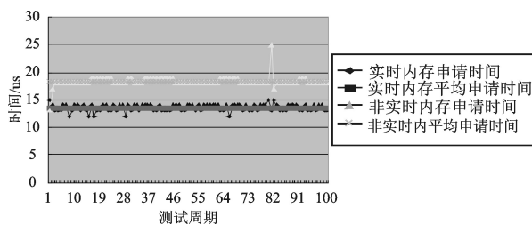
图 3 申请 4 kb 内存效率对比图
