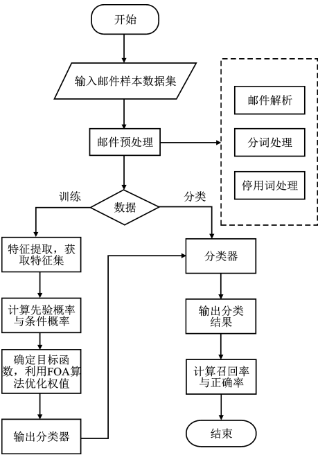
图1 FOA-NB 算法流程图
