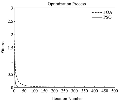
(a)迭代次数为 500
