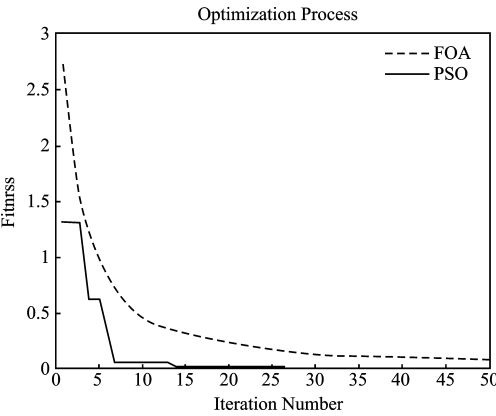
(b)迭代次数为 50
