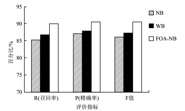
图 3 三种算法实验结果对比图
