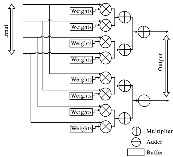
图 3 一种 CNN 卷积加速器结构
