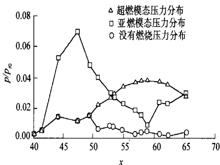
图1 超燃冲压发动机不同工作模态的压力分布
