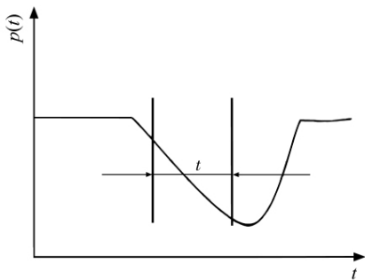
图 7 发动机喘振特征提取示意图
