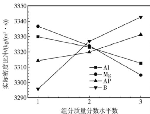
图9 不同燃料组分对实际密度比冲的影响
