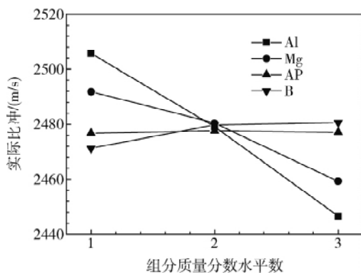
图8 不同燃料组分对发动机实际比冲的影响
