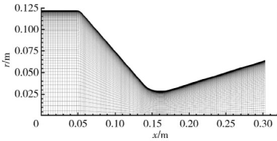
图 1 计算网格 Fig. 1 Computational mesh
