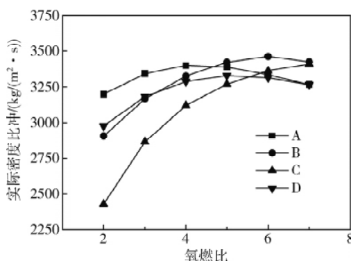
图 13 不同燃料配方的实际密度比冲
