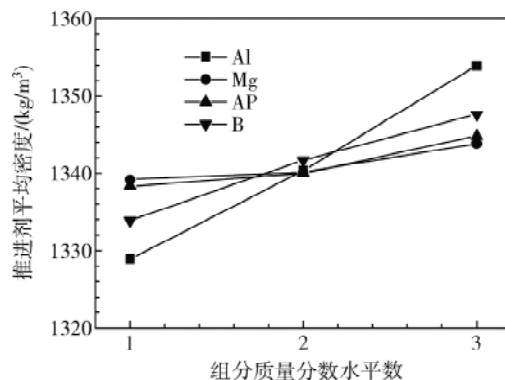
图6 不同燃料组分对推进剂平均密度的影响
