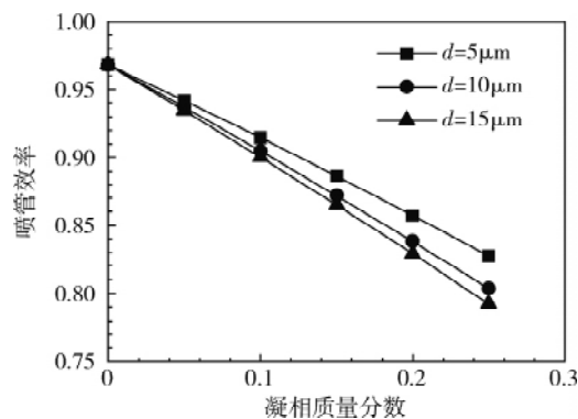
图 3 凝相参数对比冲效率的影响
