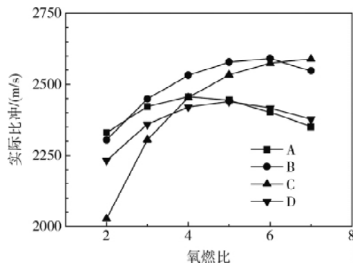
图11 不同燃料配方的实际比冲
