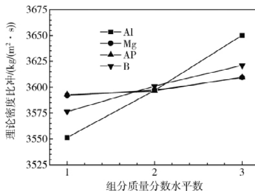
图7 不同燃料组分对理论密度比冲的影响
