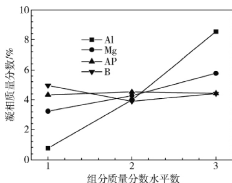
图4 不同燃料组分对凝相质量分数的影响
