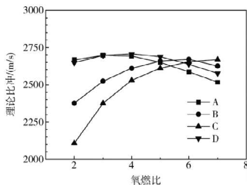
图10 不同燃料配方的理论比冲
