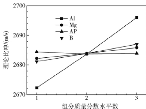
图5 不同燃料组分对理论比冲的影响
