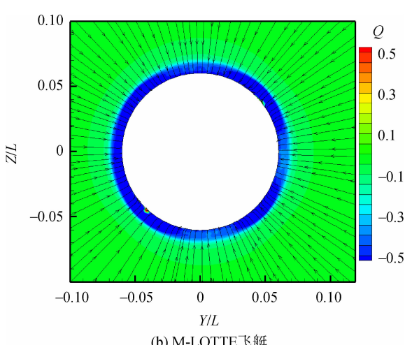
图 7 LOTTE 和 M-LOTTE 飞艇在 X/L=0.90 处截面流线和 Q 分布
