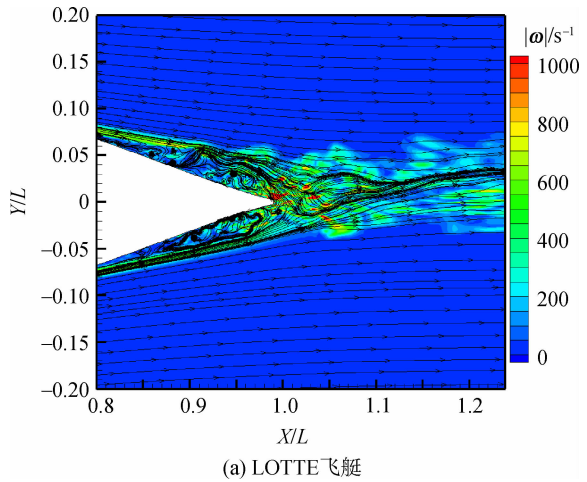
(a) LOTTE 飞艇
