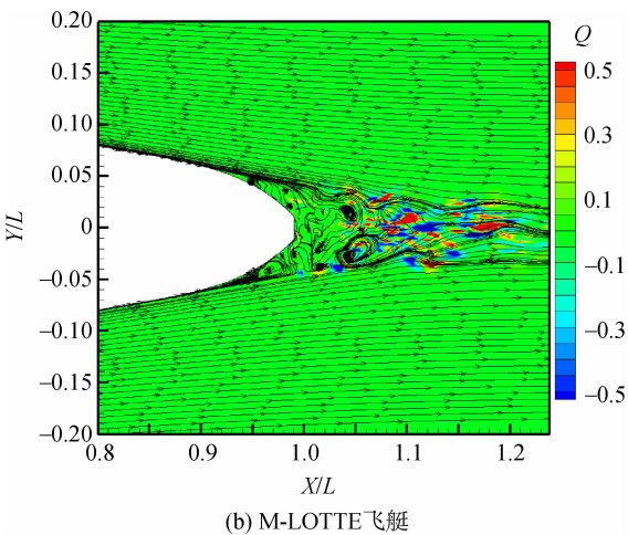
图 5 LOTTE 和 M-LOTTE 飞艇中心截面流线和 Q 分布
