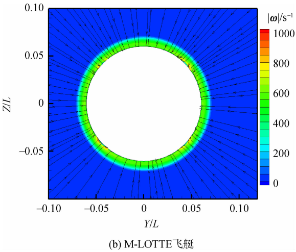
图 6 LOTTE 和 M-LOTTE 飞艇在 X/L=0.90 处截面流线和涡量分布
