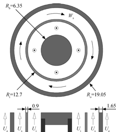
图1 分层旋流燃烧器结构示意图(单位:mm)
