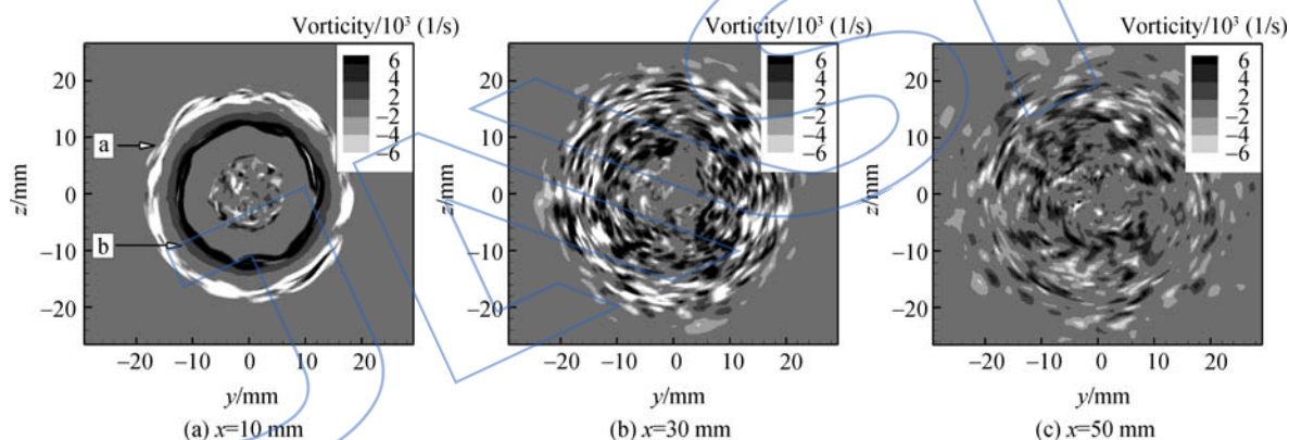
图 6 横截面上轴向涡量的云图( S_g = 0.79 )
