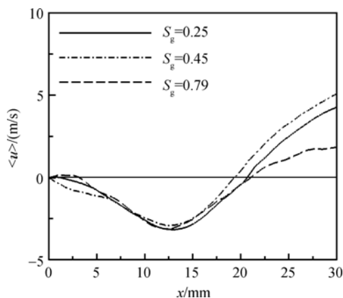
图 5 平均轴向速度沿中轴线的分布
