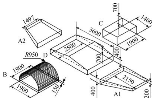
图 4 燃油系统的油箱结构(单位: mm)
