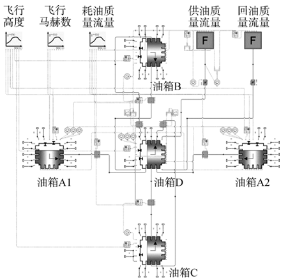
图 5 Flowmaster 中的燃油系统仿真模型
