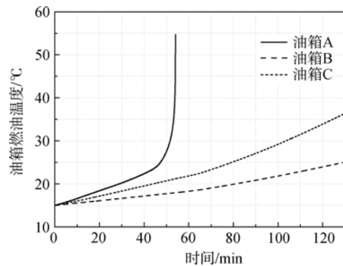
图8 油箱燃油温度
