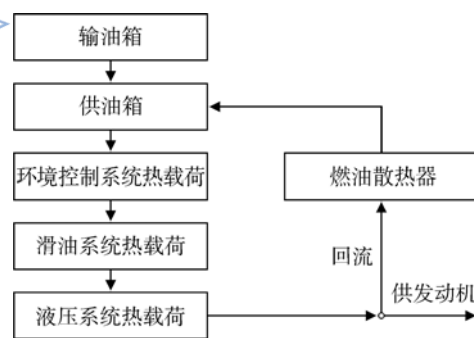
图2 综合热管理系统框图
