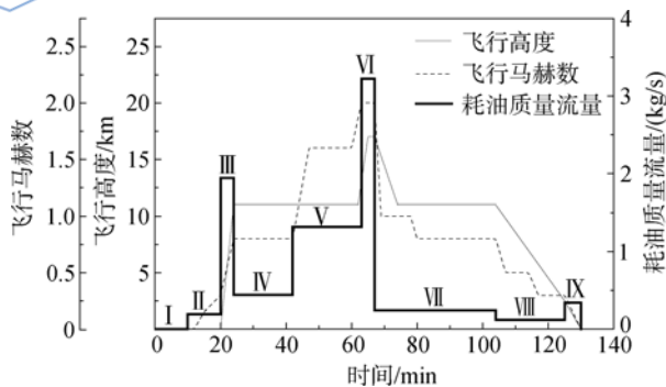
图 6 飞行剖面
