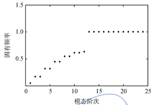
图 11 固有频率( k_c=42.6 )
