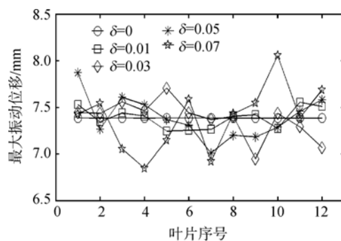
(b) 第13阶共振响应
