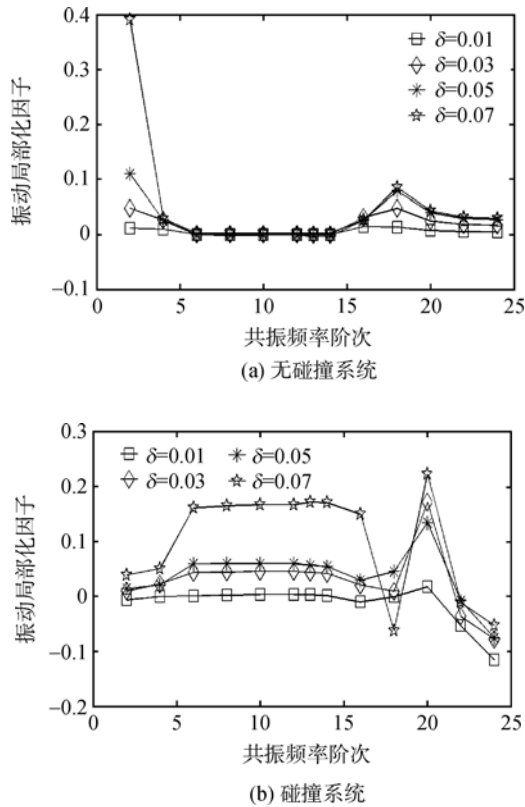
图 9 叶片刚度失谐的叶片振动局部化因子( k_c=426 )
