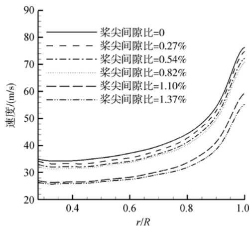
图7 涵道唇口横向截面速度分布图
