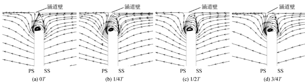
图9 1.10%桨尖间隙比下桨尖间隙流线图
