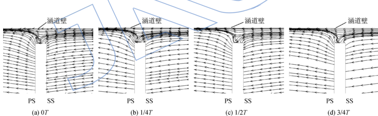
图8 0.82%桨尖间隙比下桨尖间隙流线图
