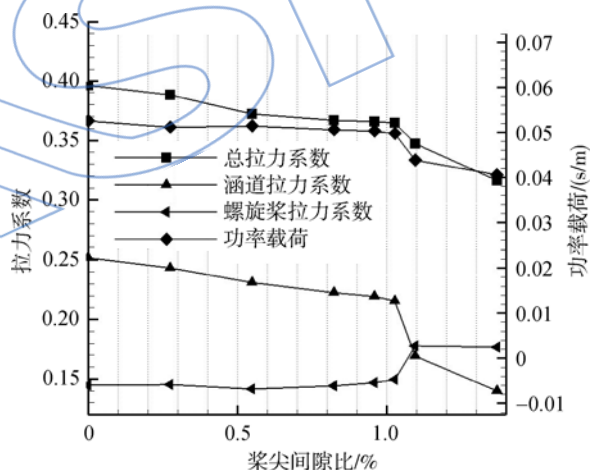
图6 涵道风扇气动力随桨尖间隙比变化图
