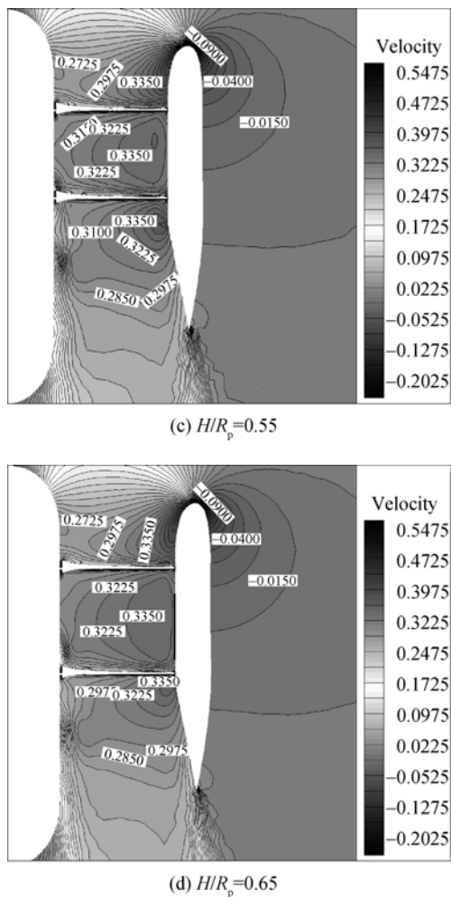
图12 不同双桨间距下中垂面上的轴向速度云图 Fig. 12 Axial velocity contour on the mid-plane at various propeller separation space
