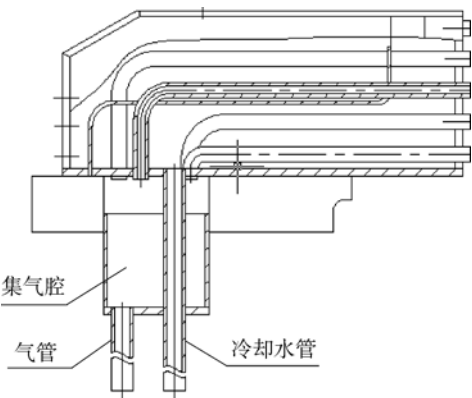
图 2 取样器结构图 Fig. 2 Structure of sampler
