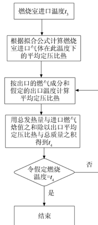
图 1 平均定压比热法计算燃烧温度流程图
