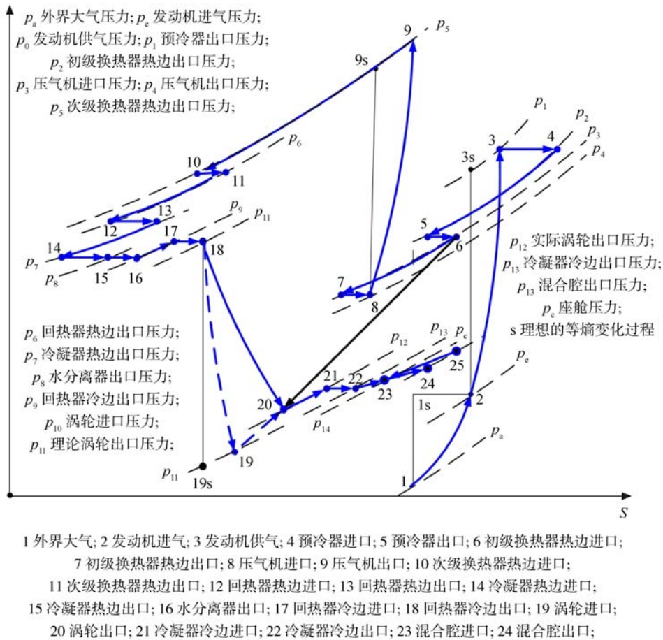
图2 空调系统空气热力过程 T-S 图
