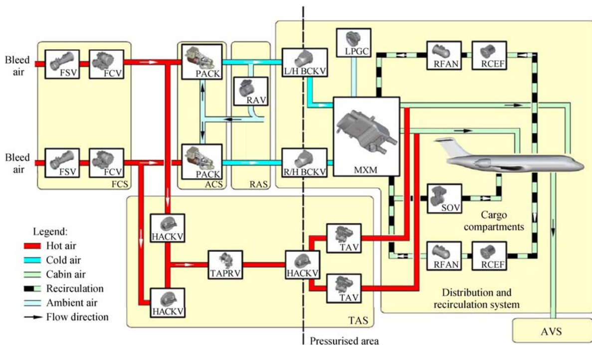
图1 空调系统示意图
