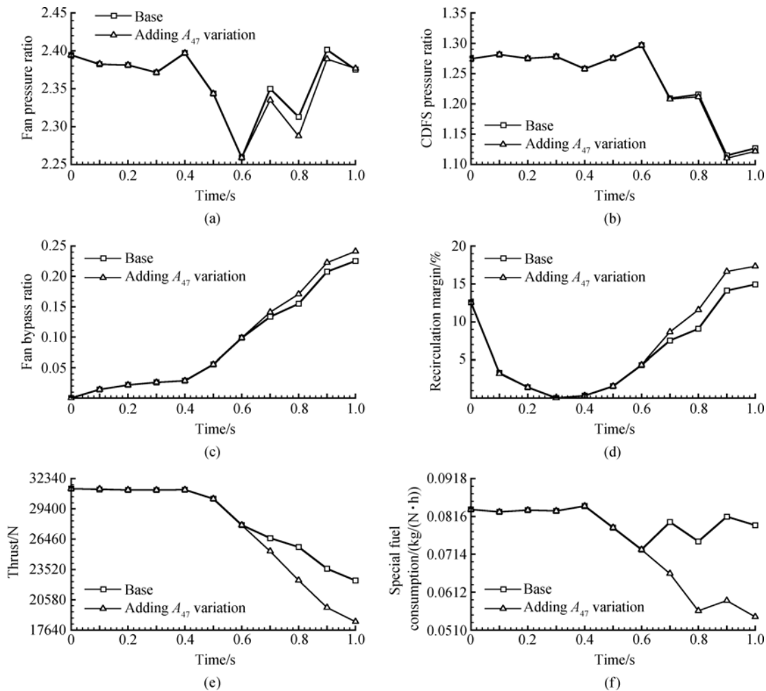
图6 单外涵至双外涵模态变循环发动机工作参数变化
