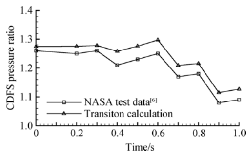
图 4 单外涵至双外涵模态 CDFS 压比对比
