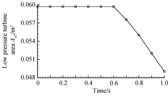
图5 单外涵至双外涵模态 A_{47} 调节规律
