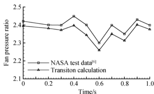
图 3 单外涵至双外涵模态风扇压比对比
