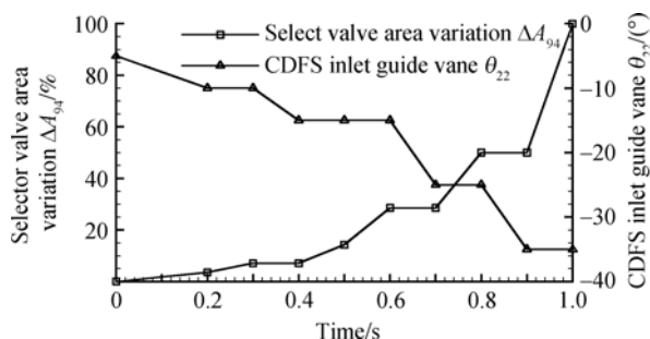
图 2 单外涵至双外涵模态几何调节规律
