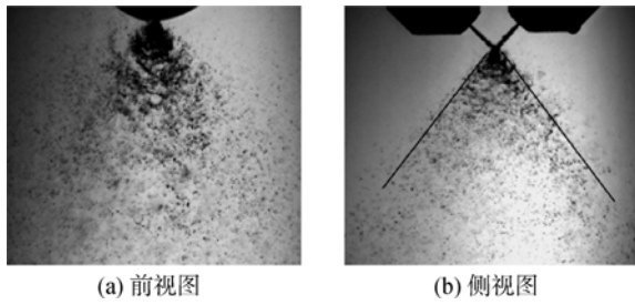
图 8 w_c = 0.15\% 的卡波姆凝胶在 U_{jet} = 28.9 \text{ m/s} 和 Re_{gen} = 9755 时的液膜破碎图像
