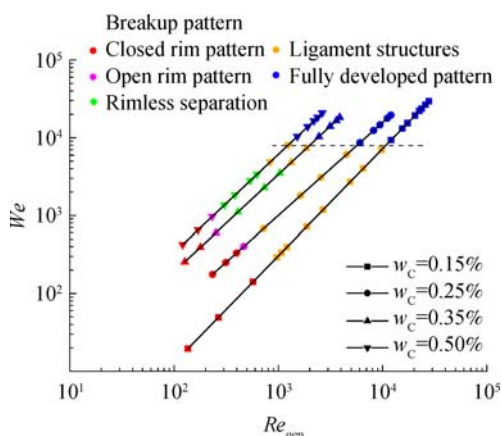
图7 4种卡波姆凝胶破碎模式图
