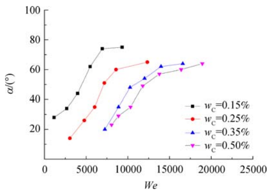
图 9 4 种不同 w_c 卡波姆凝胶的喷雾锥角随 We 的变化曲线
