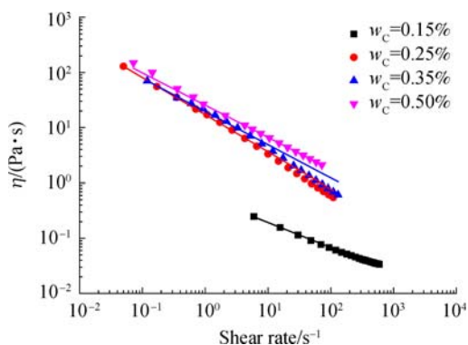
图3 4种卡波姆凝胶的流变特性曲线
