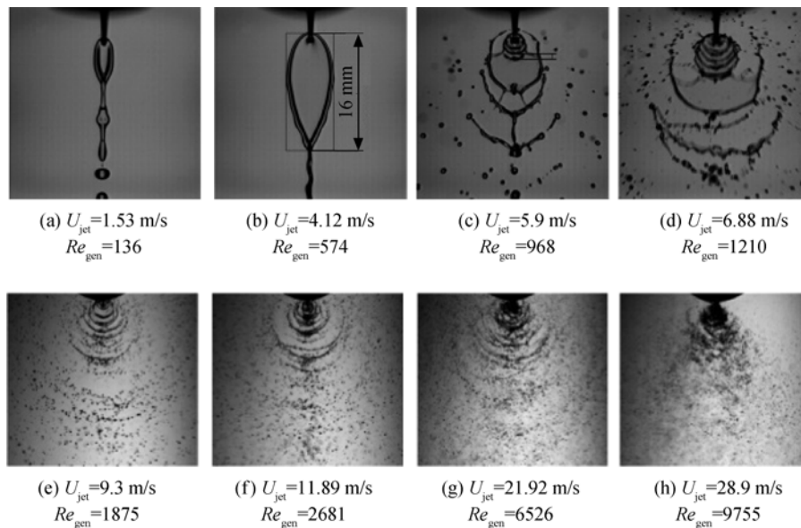
图 4 \omega_c = 0.15\% 的卡波姆凝胶撞击射流液膜破碎图像
