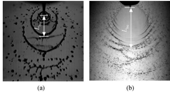
图 10 破碎长度的测量方法
