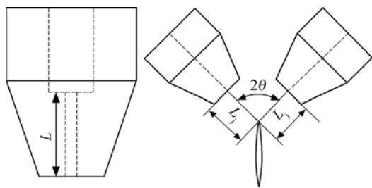
图2 喷嘴与撞击射流液膜的结构
