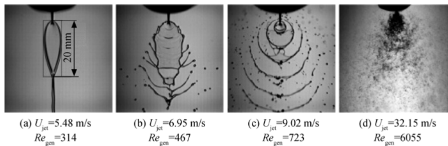
图 5 \omega_c = 0.25\% 的卡波姆凝胶撞击射流液膜破碎图像
