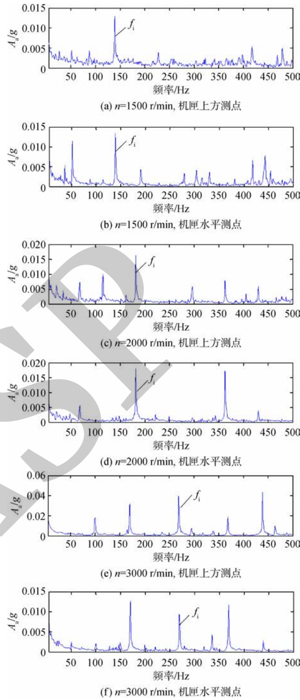
图 15 不同转速和测点下的包络谱
