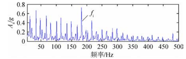
图 9 轴承座信号包络谱
