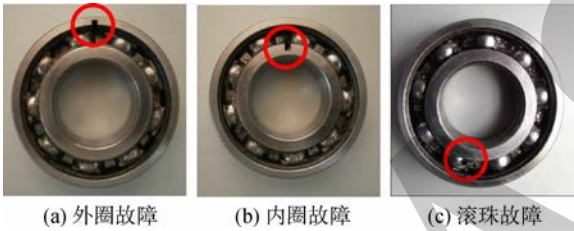
图 3 故障加工后的滚动轴承
