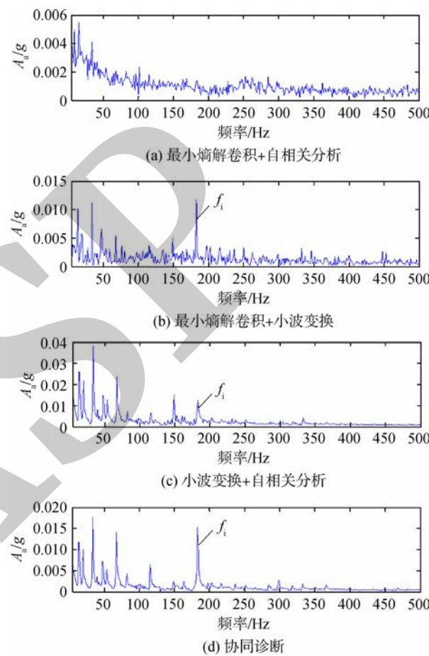
图 8 不同方法的包络谱对比
