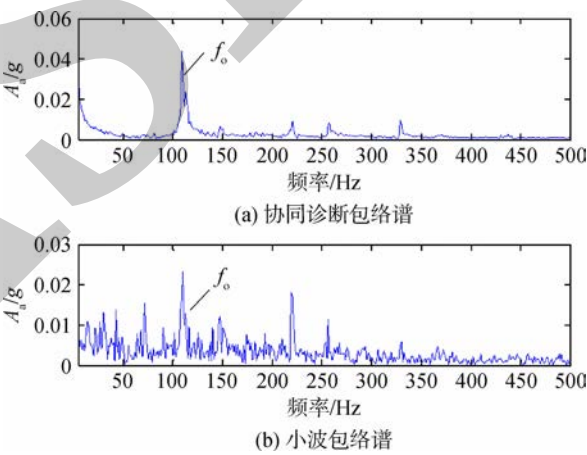
图 5 外圈故障结果对比
