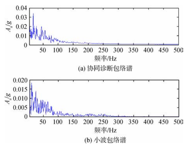
图 7 正常情况结果对比
