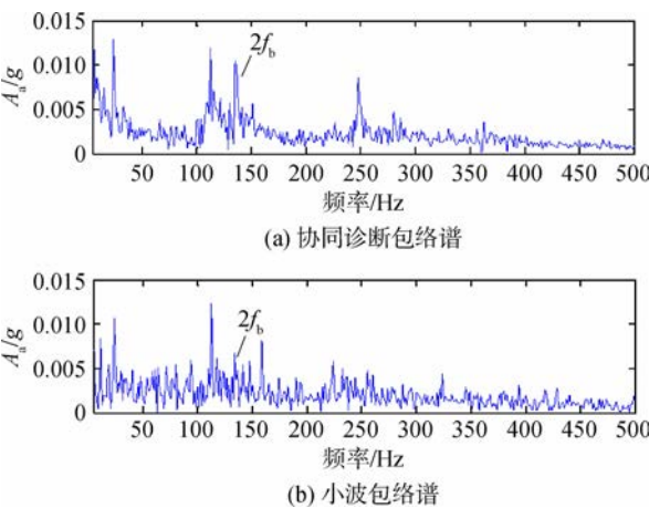
图 6 滚珠故障结果对比
