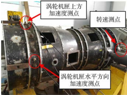
(b) 实物图(外部)
