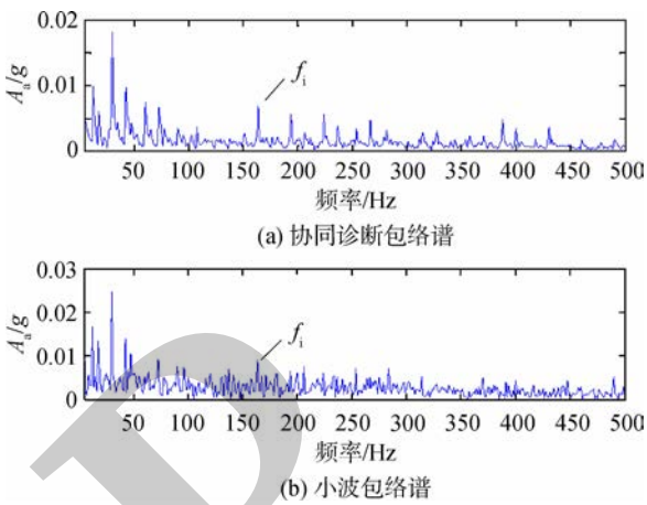
图 4 内圈故障结果对比
