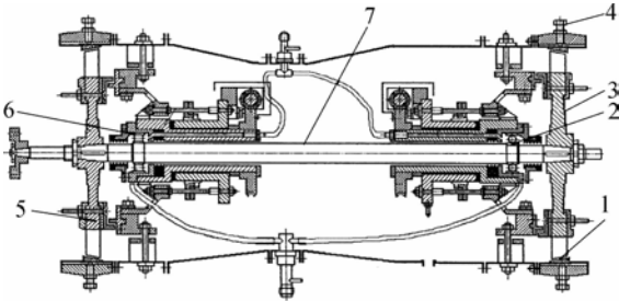
1 碰摩环;2 球轴承;3 涡轮盘;4 碰摩环点变形顶螺栓;5 压气机轮盘;6 滚柱轴承;7 轴。
