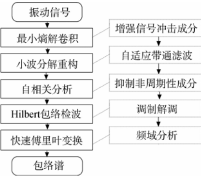
图 1 协同诊断方法流程图
