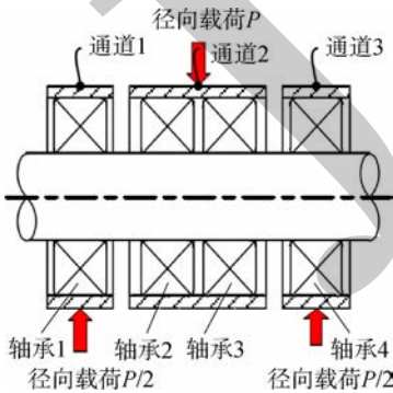
图 11 ABLT-1A 试验机加载示意图
