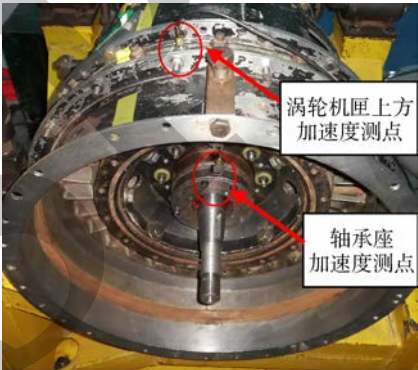
(a) 实物图(内部)
