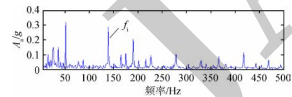
图 14 轴承座信号包络谱
