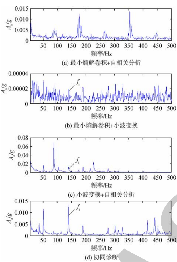
图 13 不同方法的包络谱对比
