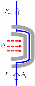
图 1 再生主动冷却
