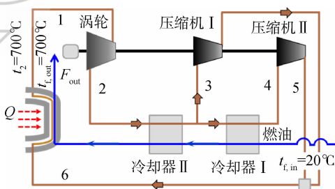
图 5 部分冷却再压缩的 S- \text{CO}_2 布雷顿循环一体化系统
