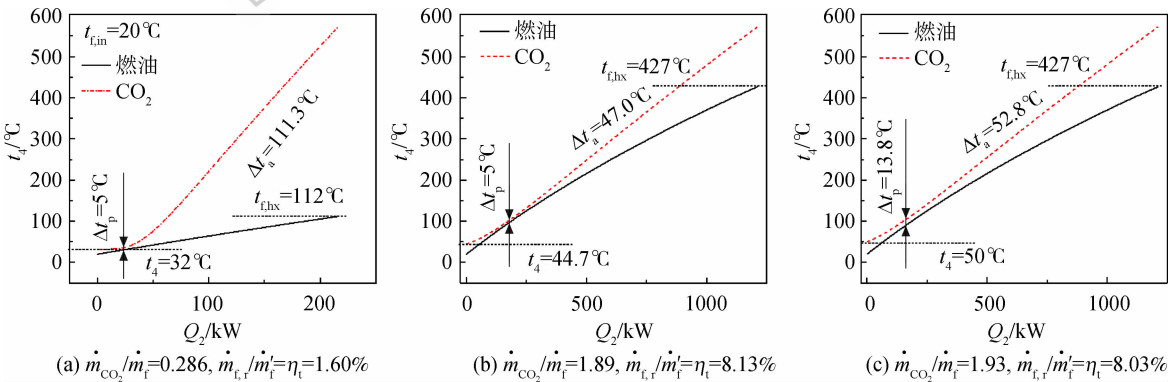
图 6 不同 CO 2 气体冷却器出口温度下沿 CO 2 流动方向的 t - Q 图
