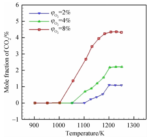
图 17 不同氧气体积分数下 \text{CO}_2 的摩尔分数图 Fig. 17 Mole fraction of \text{CO}_2 under different oxygen volume fractions
