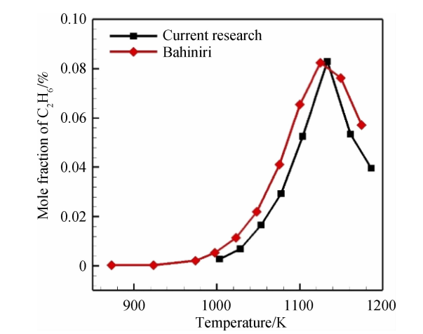
图 3 甲烷氧化实验中 C 2 H 6 的摩尔分数图 Fig. 3 Mole fraction of C 2 H 6 during methane oxidation
