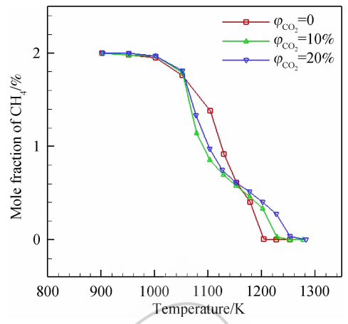
图 19 不同二氧化碳体积分数下 \text{CH}_4 的摩尔分数图 Fig. 19 Mole fraction of \text{CH}_4 under different carbon dioxide volume fractions
