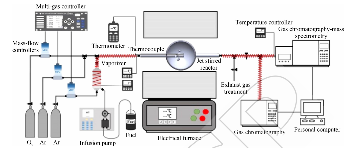
图 1 射流搅拌反应器简图 Fig. 1 Schematic diagram of jet stirred reactor
