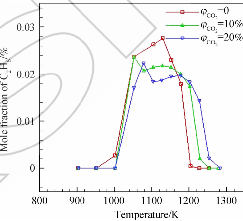
图 20 不同二氧化碳体积分数下 \text{C}_2\text{H}_6 的摩尔分数图 Fig. 20 Mole fraction of \text{C}_2\text{H}_6 under different carbon dioxide volume fractions
