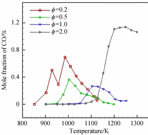
图 12 不同当量比下 CO 的摩尔分数图 Fig. 12 Mole fraction of CO under different equivalence ratios
