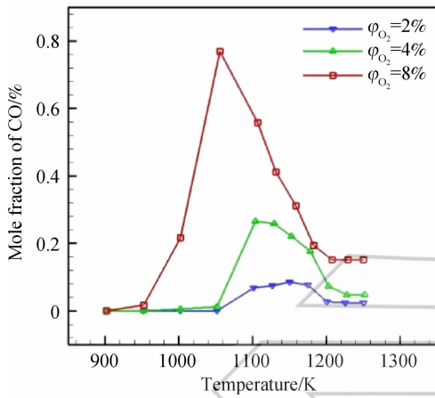
图 18 不同氧气体积分数下 \text{CO} 的摩尔分数图 Fig. 18 Mole fraction of \text{CO} under different oxygen volume fractions
