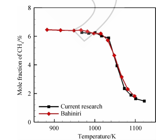
图 2 甲烷氧化实验中 CH 4 的摩尔分数图 Fig. 2 Mole fraction of CH 4 during methane oxidation
