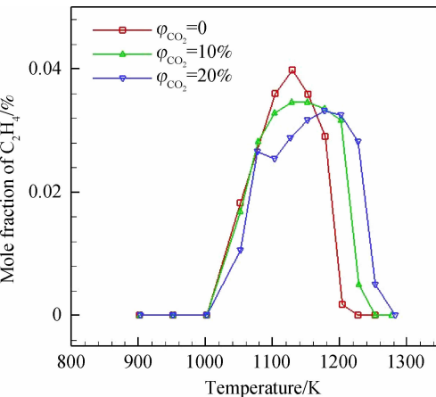
图 21 不同二氧化碳体积分数下 \text{C}_2\text{H}_4 的摩尔分数图 Fig. 21 Mole fraction of \text{C}_2\text{H}_4 under different carbon dioxide volume fractions
