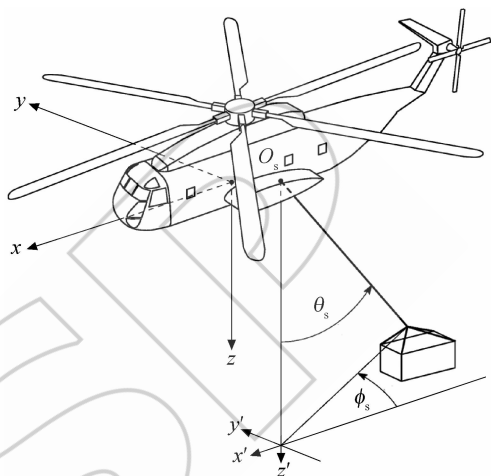
图 1 直升机吊挂耦合系统构型图
