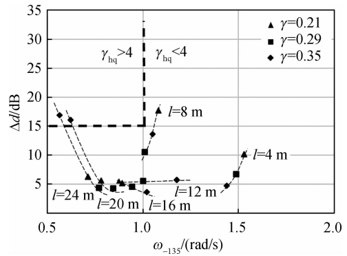
图 7 不同吊挂参数下摆角滞后反馈控制系统的飞行品质 Fig. 7 Flying qualities of slung load parameters in lagged cable angle feedback system
