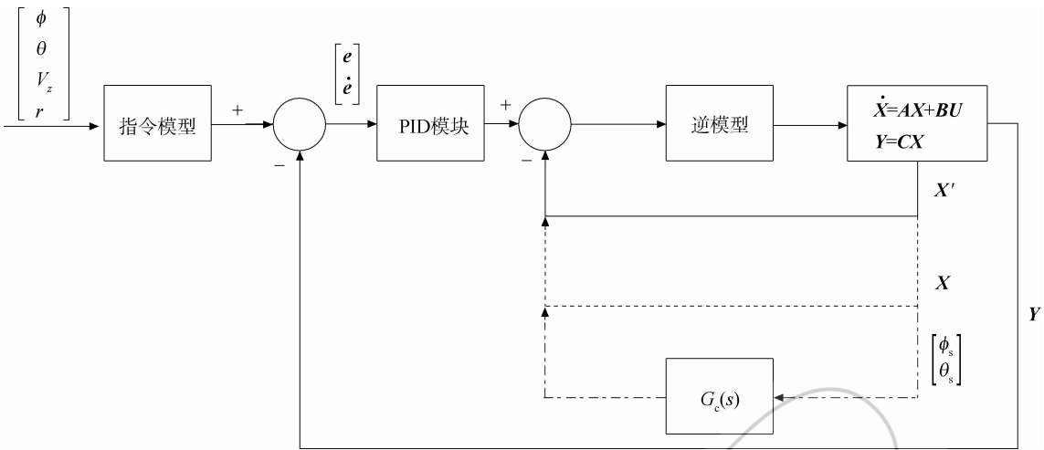
图 2 控制系统结构图
