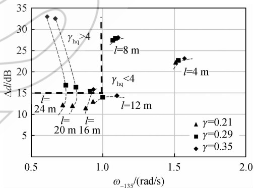
图 6 不同吊挂参数下基准控制系统的飞行品质 Fig. 6 Flying qualities of slung load parameters in basic control system
