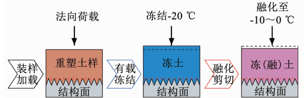
图 2 试验过程示意
