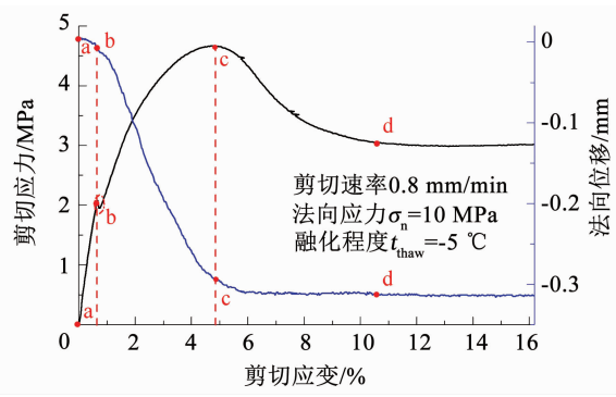
图5 剪切应力和法向位移特征曲线 ( \sigma_n = 10\text{ MPa} 、 t_{\text{thaw}} = -5\text{ }^{\circ}\text{C} )
