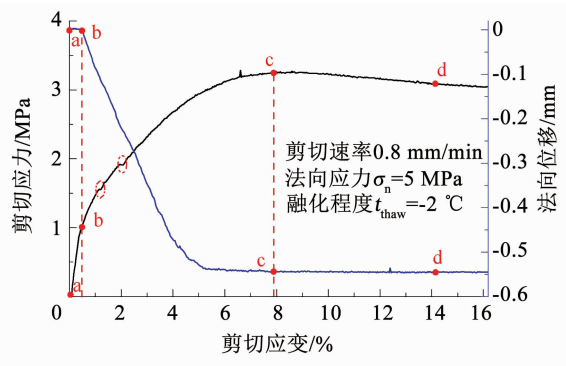
图6 剪切应力和法向位移特征曲线 ( \sigma_n = 5\text{ MPa} 、 t_{\text{thaw}} = -2\text{ }^{\circ}\text{C} )
