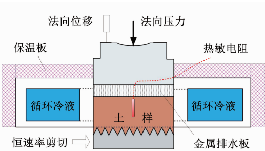
图 3 试样温度量测与控制
