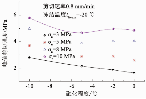
图8 峰值剪切强度与融化程度对应关系
