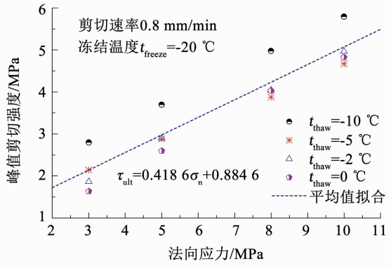
图7 峰值剪切强度与法向应力对应关系
