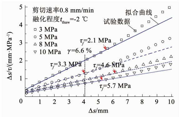
图 9 融化程度 -2 °C 时 \gamma/\tau - \gamma 关系拟合曲线
