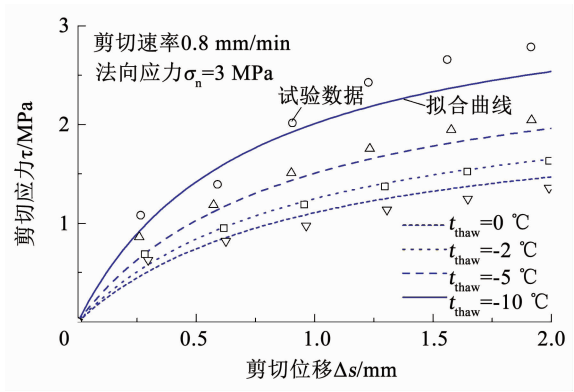
图 10 3 MPa 应力下剪切应力-应变拟合曲线 ( \tau < \tau_f )
