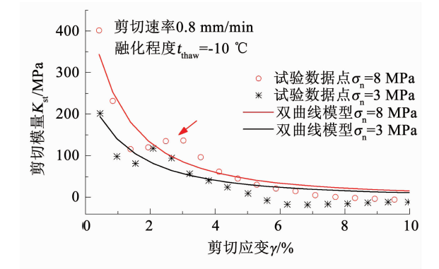
图 12 接触面剪切模量变化趋势 Fig. 12 Trends of shear modulus of interface
