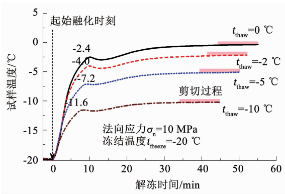
图 4 试验中试样温度曲线
