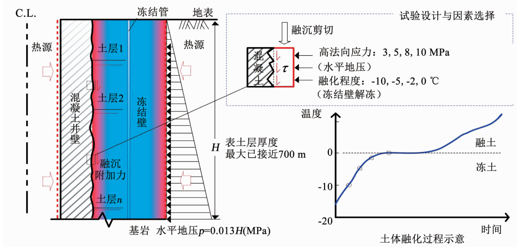
图1 试验设计思路 Fig. 1 Design of test
