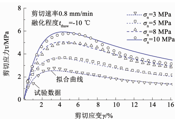
图 13 -10\text{ }^{\circ}\text{C} 条件下剪切应力-位移拟合曲线
