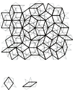
图 3 紧缩法则前后的彭罗斯单元的相互关系
