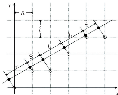
图 5 一维准晶的直接投影示意图
