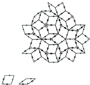
图 4 彭罗斯拼砌的一种匹配法则
