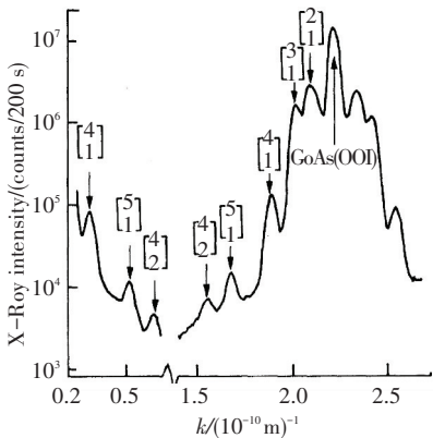
图 2 一维准晶的 X 射线衍射 [29]
