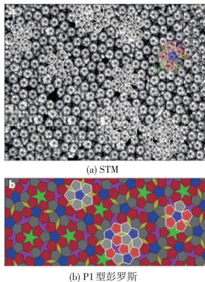
图 1 Au(1,1,1) 表面二茂铁甲酸的 STM 图与对应的 P1 型彭罗斯图 [22]
