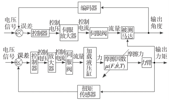
图 5 摩擦加载系统原理方框图
