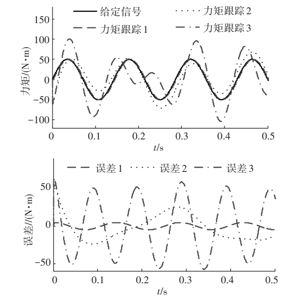
图 2 传统电液负载模拟器力矩仿真
