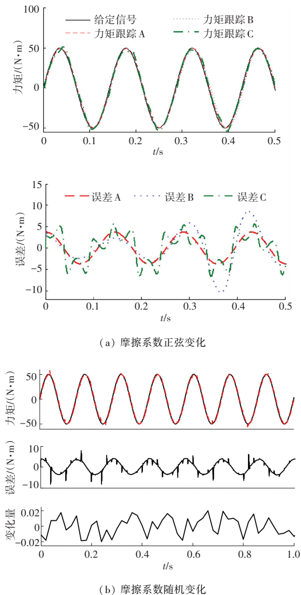
图 6 摩擦系数变化时的力矩跟踪仿真
