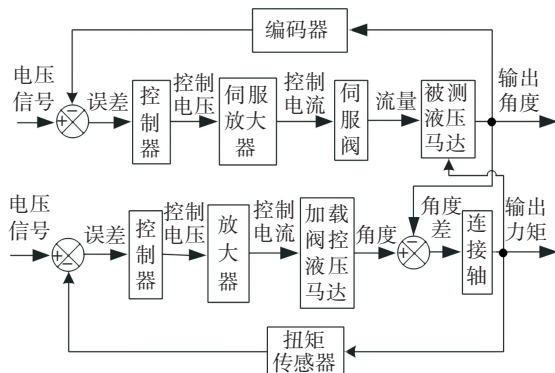
图 1 传统电液负载模拟器原理框图
