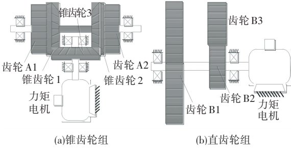
图 4 摩擦加载系统换向机构
