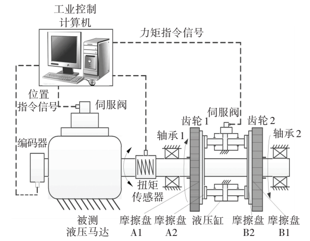
图 3 摩擦电液加载系统原理
