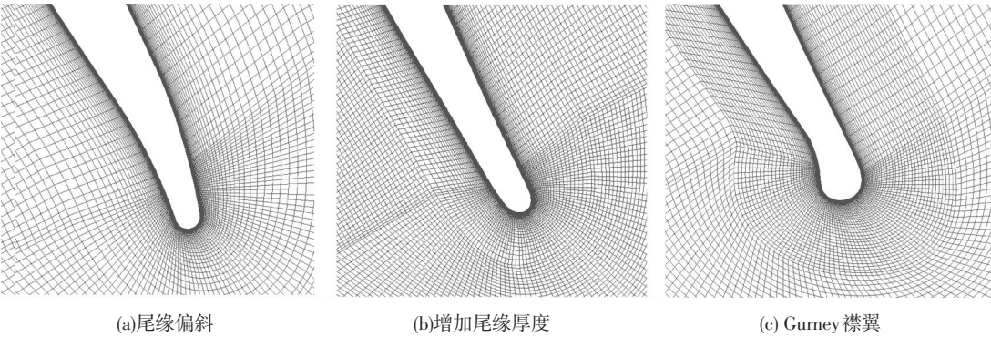
图 2 尾缘处计算网格
