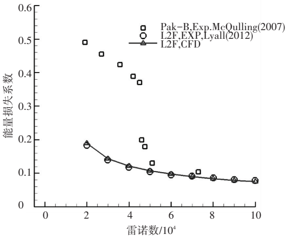
图 4 雷诺数对能量损失系数的影响
