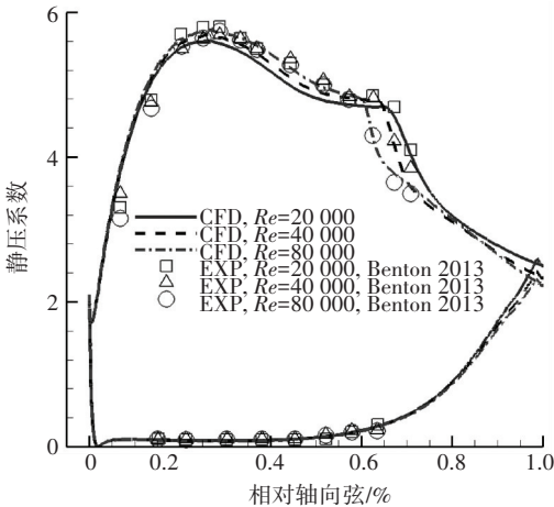
图 3 静压系数分布
