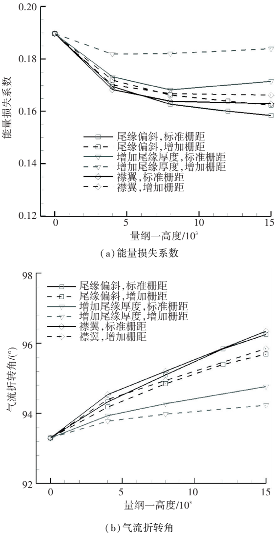
图 10 Re=20\ 000 时量纲一高度对能量损失系数和气流折转角的影响
