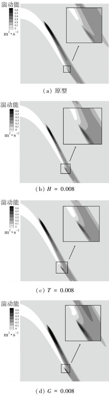
图 9 Re=20\ 000 时湍动能分布
