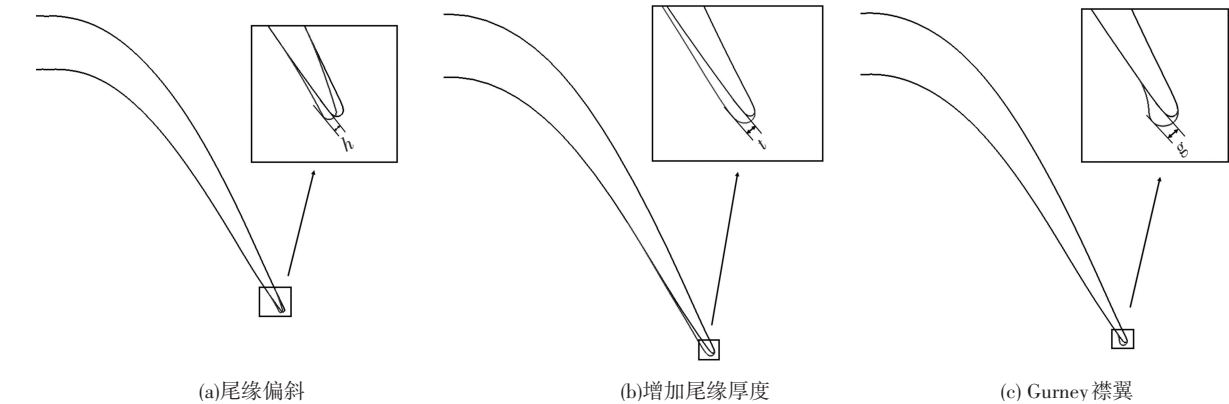
图 1 尾缘形状示意
