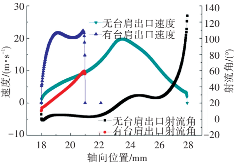
图 9 开口 1 mm 的出口速度和射流角曲线
