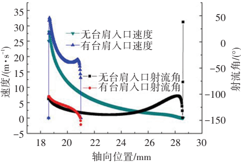
图 10 开口-1.6 mm 的入口速度和射流角曲线
