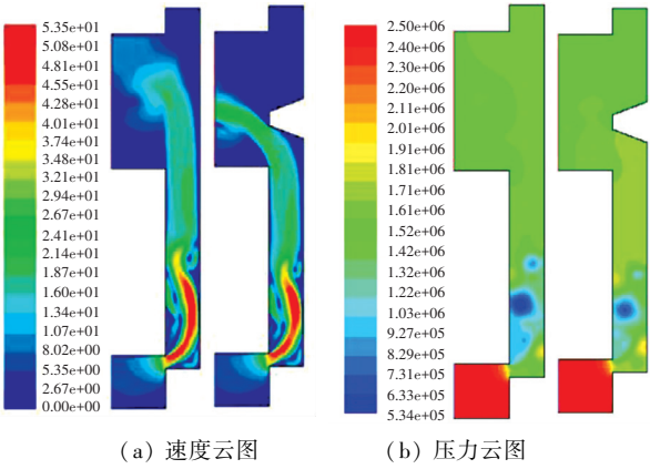
图 4 开口 1 mm 流场
