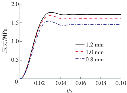
图 13 改变供油孔时输出压力阶跃响应曲线
