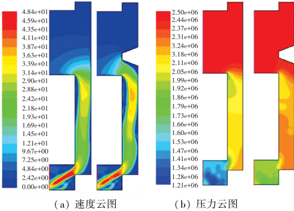
图 5 开口-1.6 mm 流场
