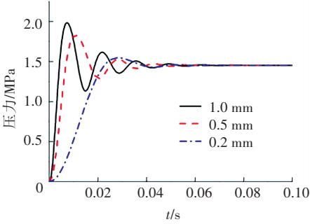
图 12 不同反馈阻尼孔时输出压力阶跃响应曲线
