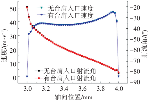
图 8 开口 1 mm 的入口速度和射流角曲线
