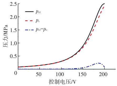
图 3 先导压力特性曲线
