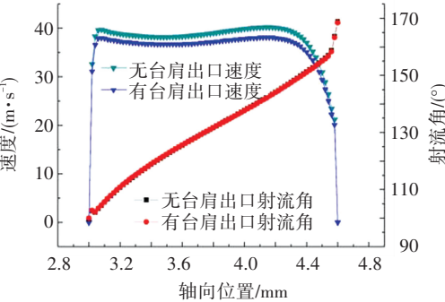
图 11 开口-1.6mm 的出口速度和射流角曲线
