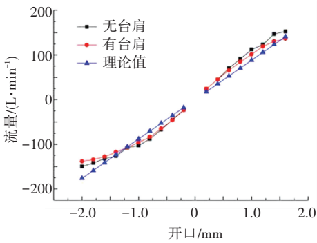
图 7 主阀流量特性
