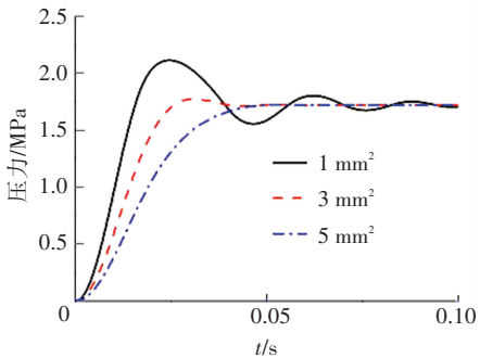
图 14 不同负载节流阀面积时输出压力阶跃响应曲线
