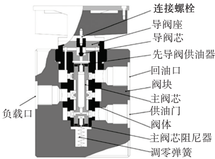
图 1 比例式减压阀结构
