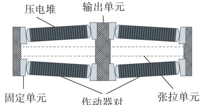
图 2 压电作动器
