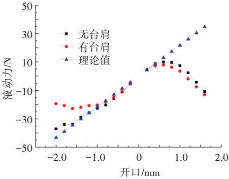
图 6 主阀液动力特性
