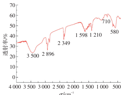
图 3 \text{Fe}_3\text{O}_4 微球的红外图谱
