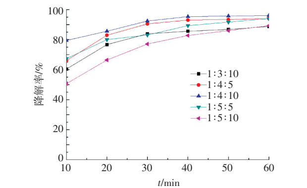
图 5 不同反应物配比时亚甲基蓝降解率
