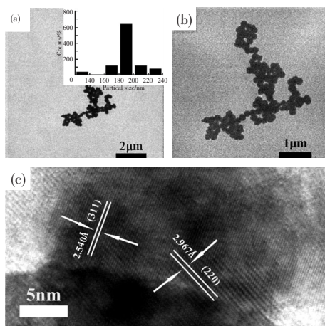
(a) 平均粒径 (200 \pm 0.5) nm 的 \text{Fe}_3\text{O}_4 微球的 TEM 图像; (b) \text{Fe}_3\text{O}_4 微球的 TEM 图像; (c) \text{Fe}_3\text{O}_4 微球的高分辨 TEM 图像
