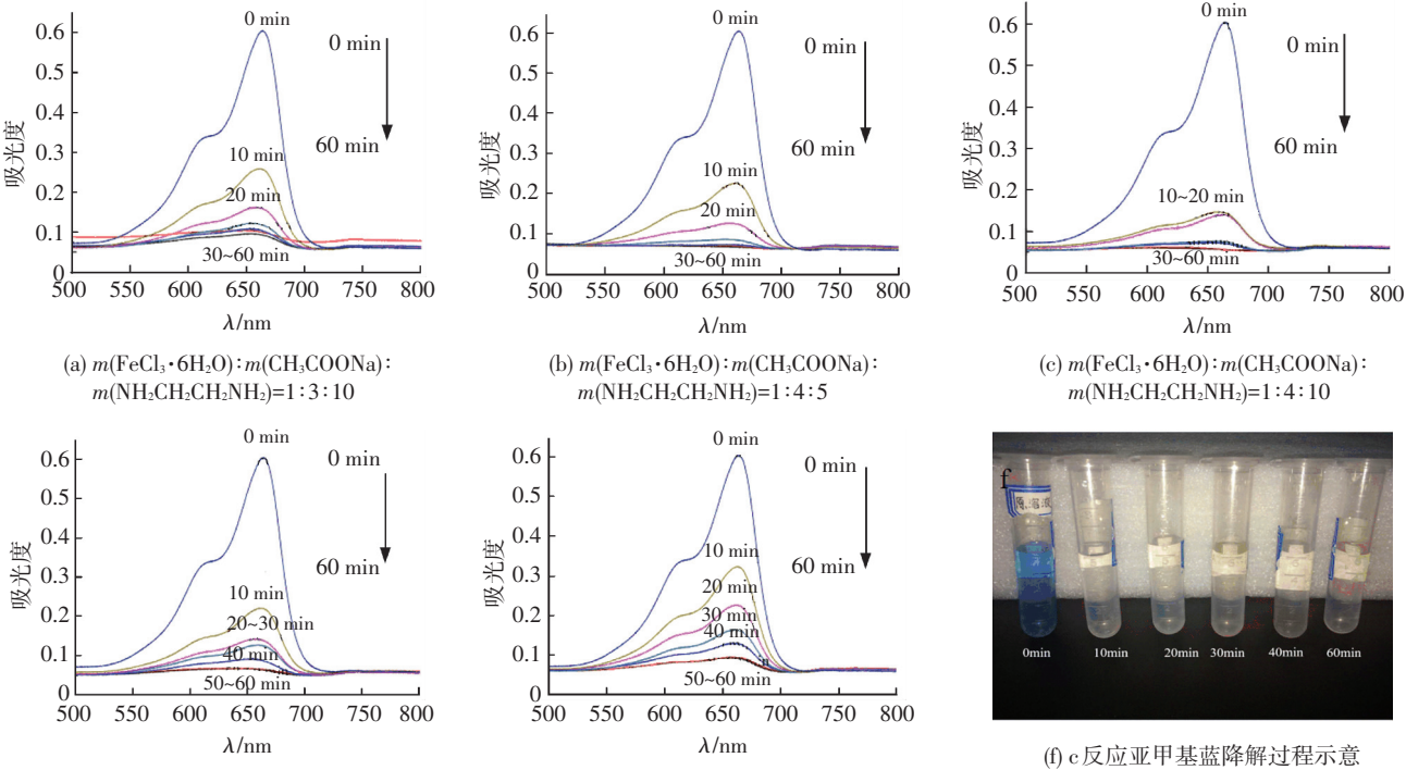
图 4 不同反应物配比所合成磁性 Fe 3 O 4 微球降解亚甲基蓝紫外-可见光谱及 c 反应亚甲基蓝降解过程实物
