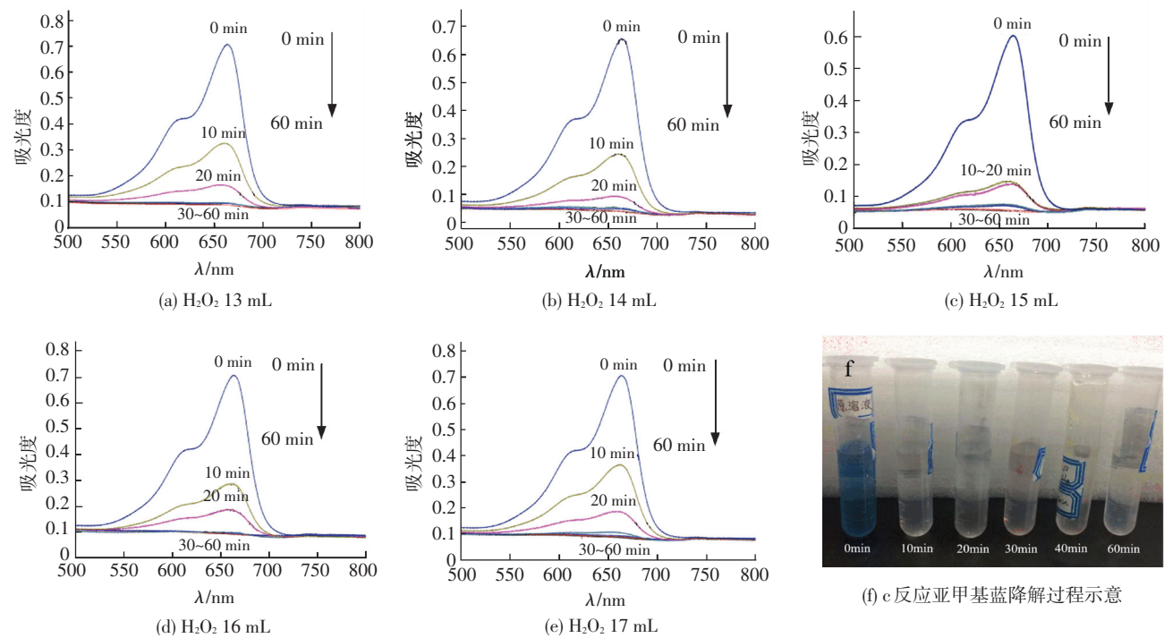
图 7 不同过氧化氢用量所合成磁性 \text{Fe}_3\text{O}_4 微球降解亚甲基蓝紫外-可见光谱及 c 反应亚甲基蓝降解过程示意
