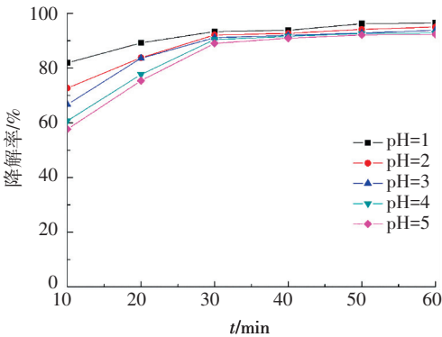
图 10 不同 pH 亚甲基蓝降解率
