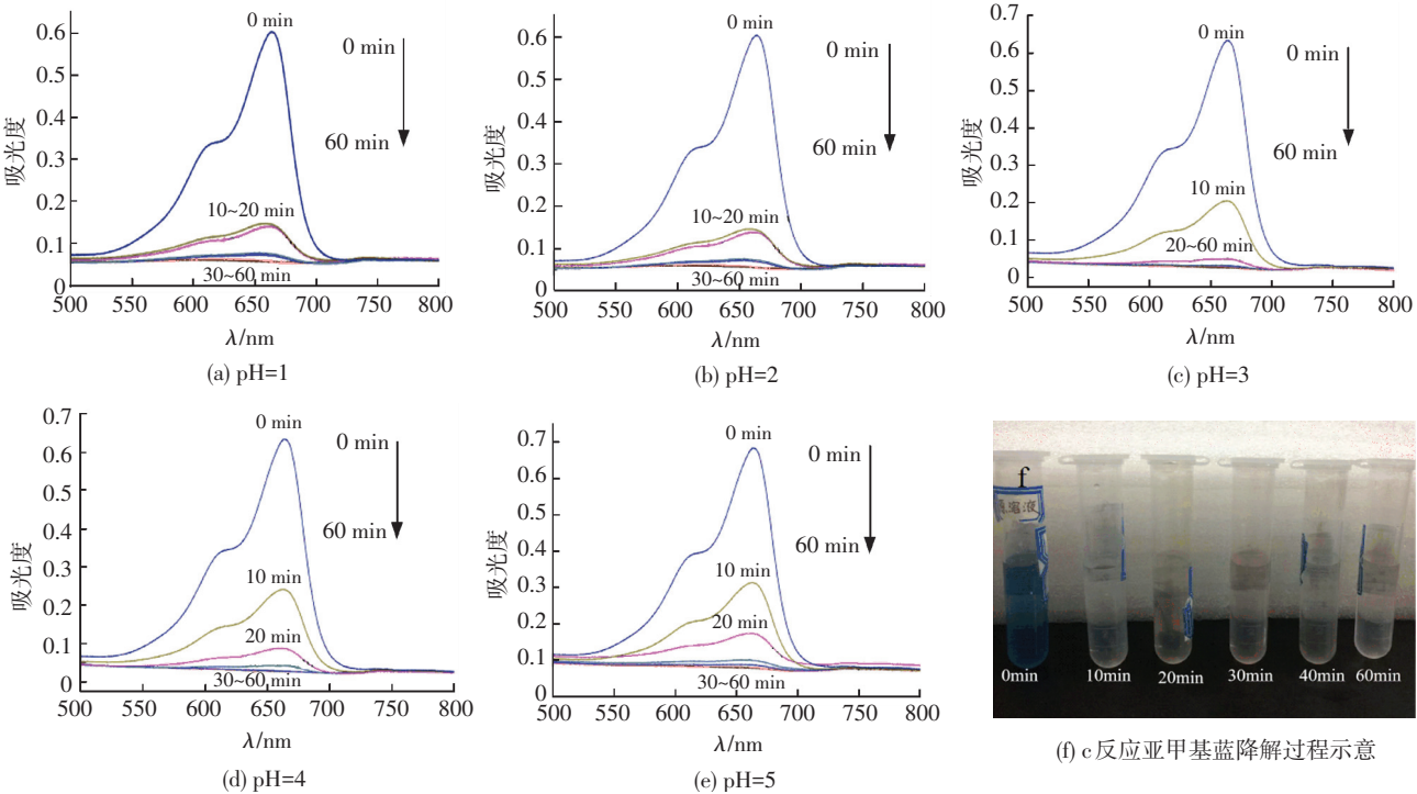
图 9 不同 pH 所合成磁性 Fe 3 O 4 微球降解亚甲基蓝紫外-可见光谱及 a 反应亚甲基蓝降解过程实物
