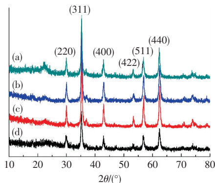
(a) m(\text{FeCl}_3 \cdot 6\text{H}_2\text{O}) : m(\text{CH}_3\text{COONa}) : m(\text{NH}_2\text{CH}_2\text{CH}_2\text{NH}_2) = 1 : 3 : 10 ; (b) m(\text{FeCl}_3 \cdot 6\text{H}_2\text{O}) : m(\text{CH}_3\text{COONa}) : m(\text{NH}_2\text{CH}_2\text{CH}_2\text{NH}_2) = 1 : 4 : 5 ; (c) m(\text{FeCl}_3 \cdot 6\text{H}_2\text{O}) : m(\text{CH}_3\text{COONa}) : m(\text{NH}_2\text{CH}_2\text{CH}_2\text{NH}_2) = 1 : 4 : 10 ; (d) m(\text{FeCl}_3 \cdot 6\text{H}_2\text{O}) : m(\text{CH}_3\text{COONa}) : m(\text{NH}_2\text{CH}_2\text{CH}_2\text{NH}_2) = 1 : 5 : 5
