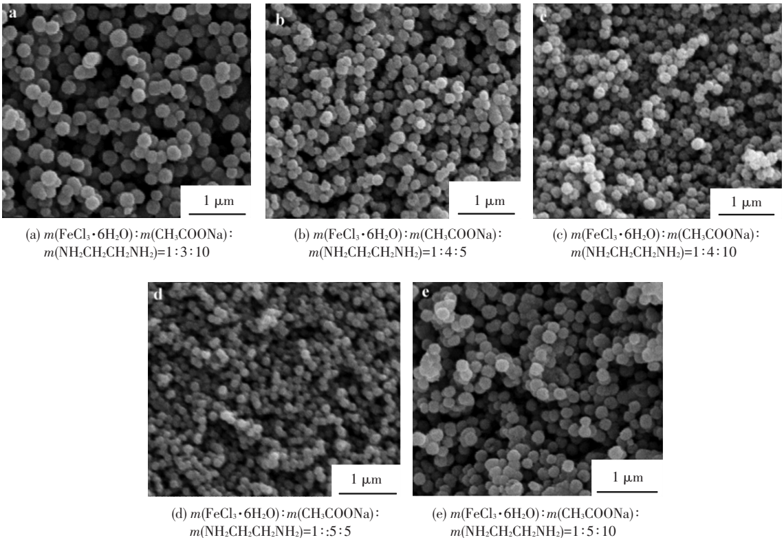
图 6 不同反应物配比所合成 \text{Fe}_3\text{O}_4 微球 SEM 图像 Fig.6 SEM picture of as-synthesized \text{Fe}_3\text{O}_4 nanospheres with different initial ratio of reactants
