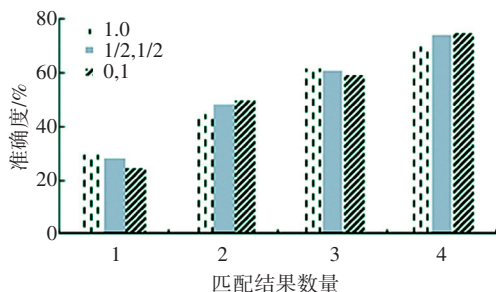
图 7 不同权重配比的准确度比较
