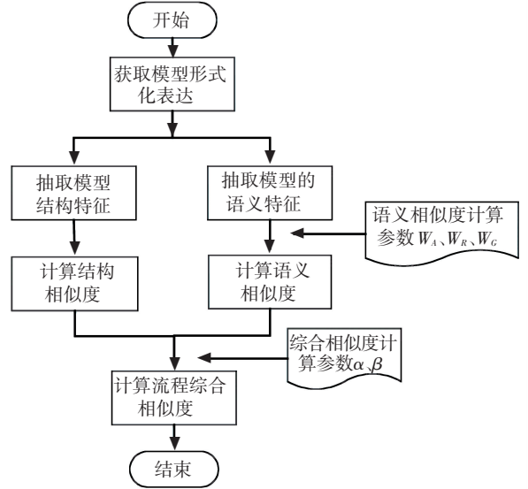
图2 相似度计算过程
