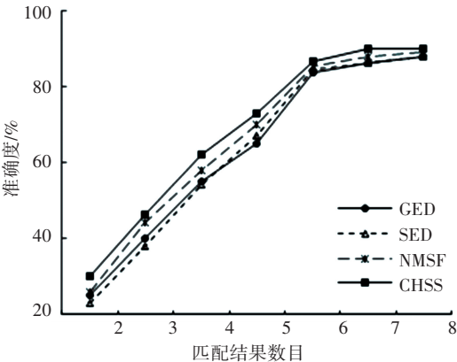
图 5 不同相似度算法准确度比较
