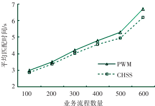
图 6 相似度算法平均匹配耗时比较
