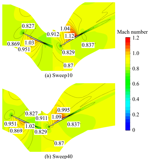
图 6 巡航状态下 50% 叶高马赫数分布 Fig. 6 Mach number distributions at 50% span at cruise condition
