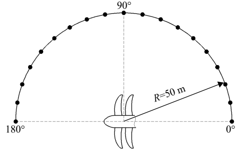
图3 虚拟麦克风布置
