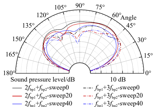
图 19 不同后掠角下前后桨干涉声压级指向性
