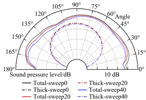
图16 不同后掠角下对转桨扇声压级指向性
