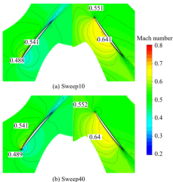
图 7 起飞状态下 50% 叶高马赫数分布 Fig. 7 Mach number distributions at 50% span at take-off condition
