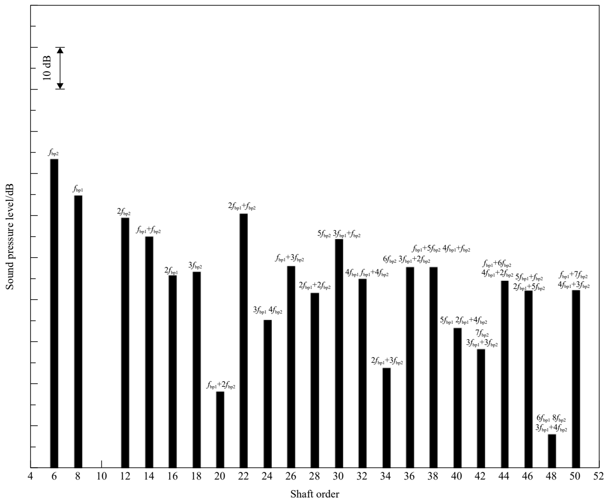
图 14 对转桨扇噪声频谱(后掠角 30°) Fig. 14 Noise spectrum of the propfan (backward sweep angle 30°)
