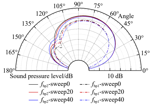
图 18 不同后掠角下桨扇桨叶通过频率的声压级指向性
