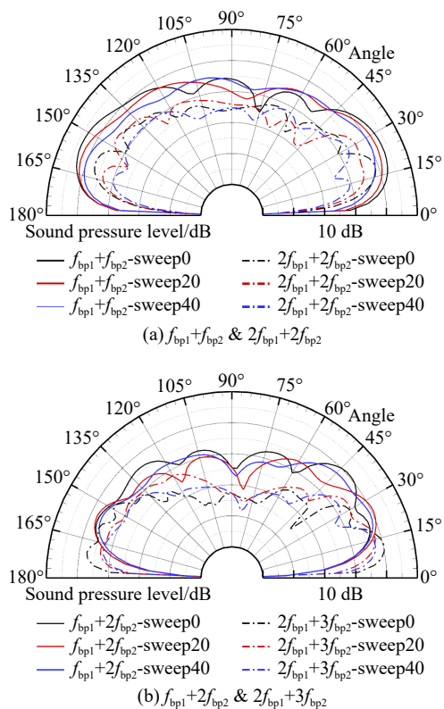
图 22 不同后掠角下前后桨干涉声压级指向性
