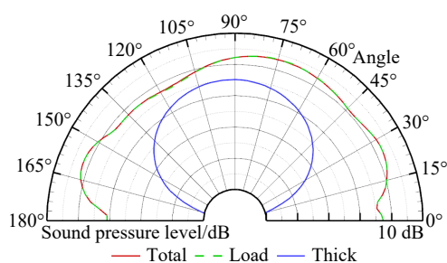
图15 对转桨扇声压级指向性(sweep30)
