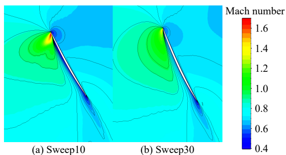
图9 起飞状态下95%叶高后桨马赫数分布
