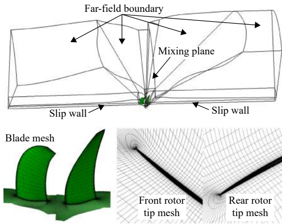
图2 计算网格及边界条件 [21]
