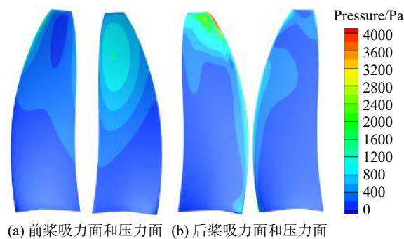
图10 起飞状态桨叶表面静压的1阶谐波
