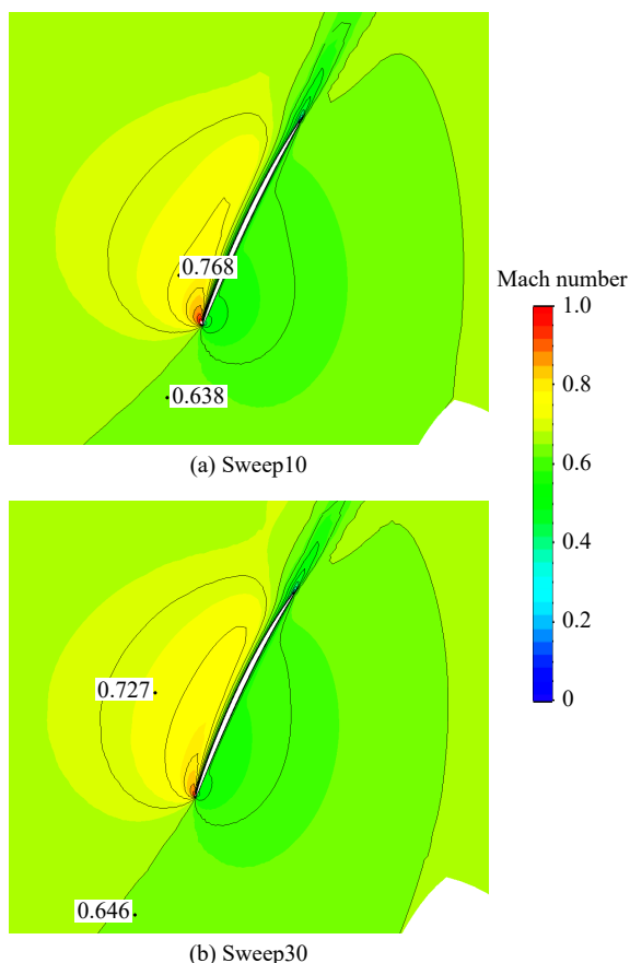
图8 起飞状态下95%叶高前桨马赫数分布
