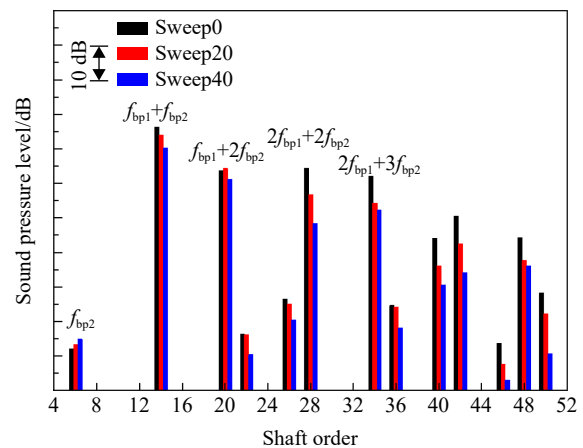
图 20 不同后掠角下 160°角向位置桨扇噪声频谱
