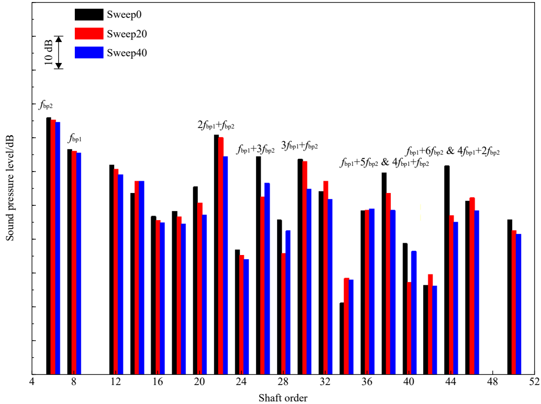
图 17 不同后掠角下 70°角向位置桨扇噪声频谱对比
