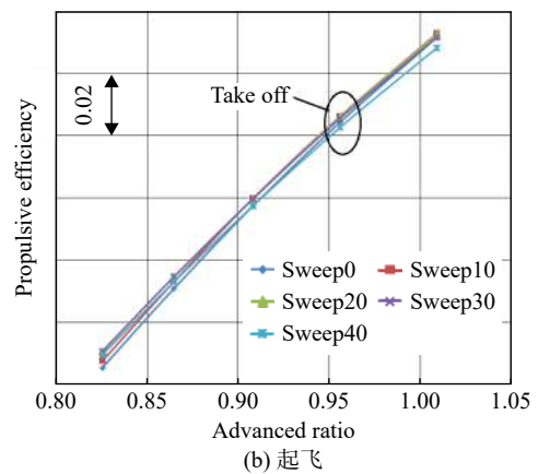
图4 桨扇巡航和起飞状态性能
