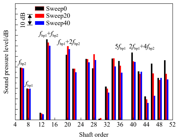
图 21 不同后掠角下 30°角向位置桨扇噪声频谱
